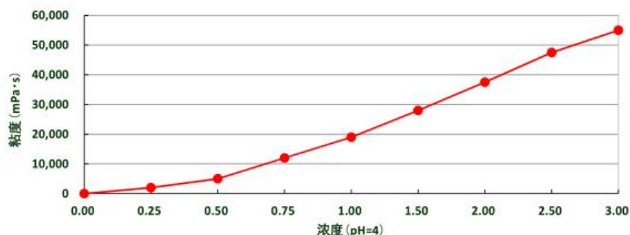
5、中和剂浓度与黏度曲线图表
